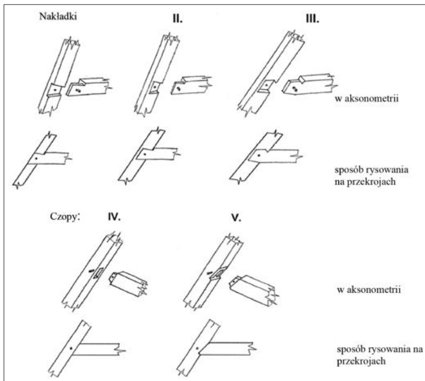
Rys. 63. Połączenia jętek z krokiewmi muszą odpowiadać rzeczywistości (rys. J. Tajchman)
