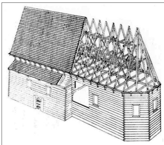
Rys. 64. Najtrudniejsze do inwentaryzacji są więzby storczykowe, czyli więzby ze słupami wiszącymi. Aksonometria na podstawie R. Brykowski, Drewniana architektura kościelna w Małopolsce XV w. , „Studia z Historii Sztuki” 1981, t. 31 (rys. J. Tajchman)
